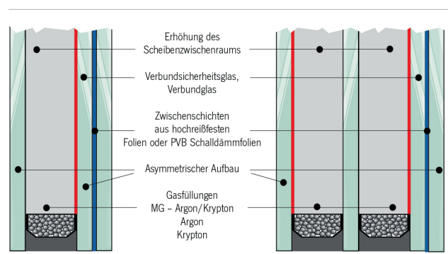
Scheibenaufbau mit PVB-Folie
